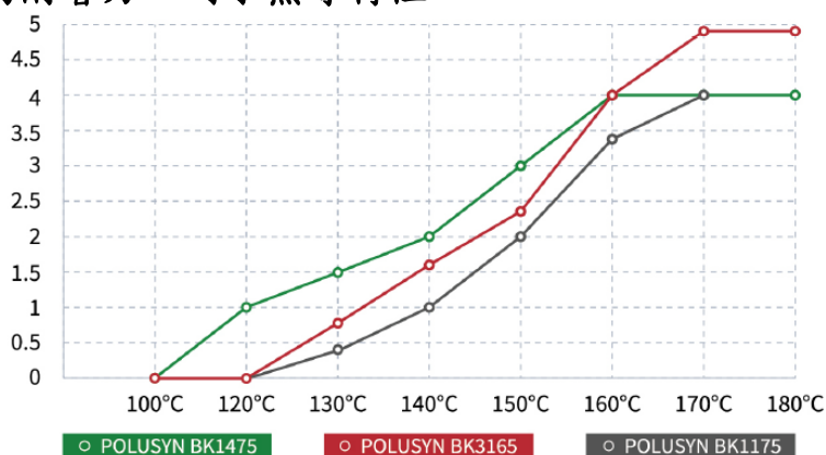
封閉型固化劑硬度與溫度之關係(30 分鐘)
